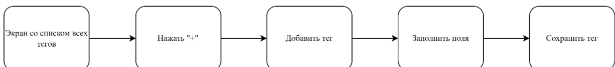
Рисунок 42 - Добавление тега
