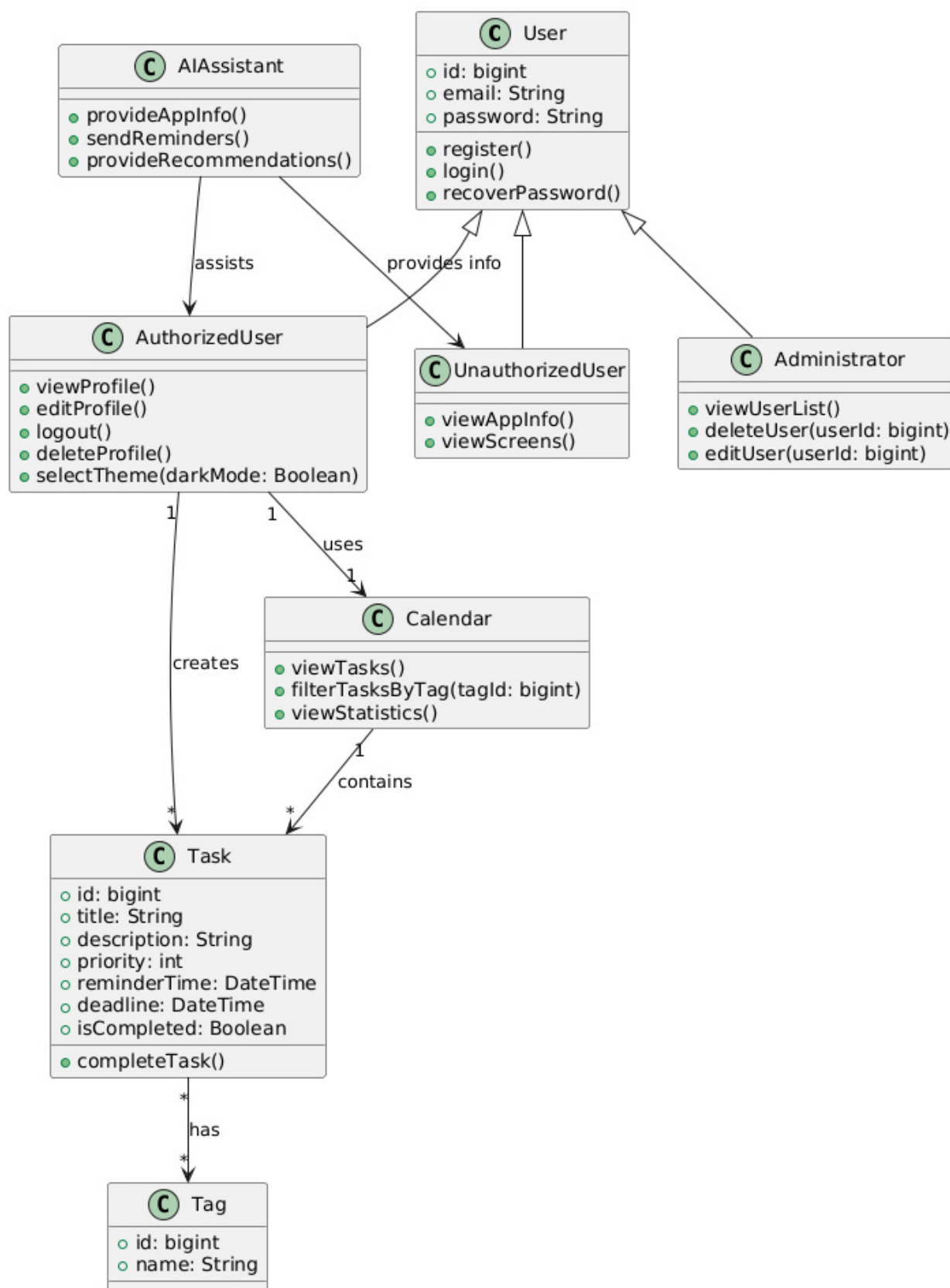
Рисунок 43 - Диаграмма классов
