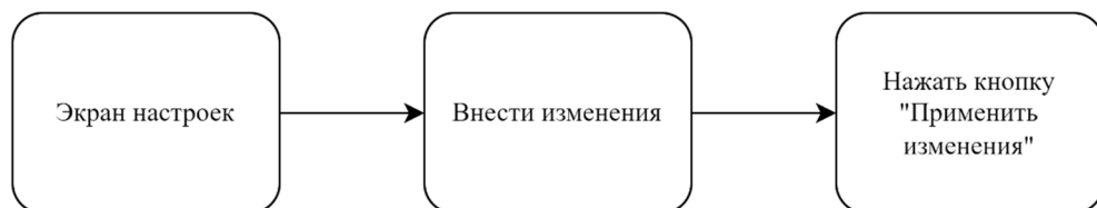
Рисунок 30 - Изменение профиля
