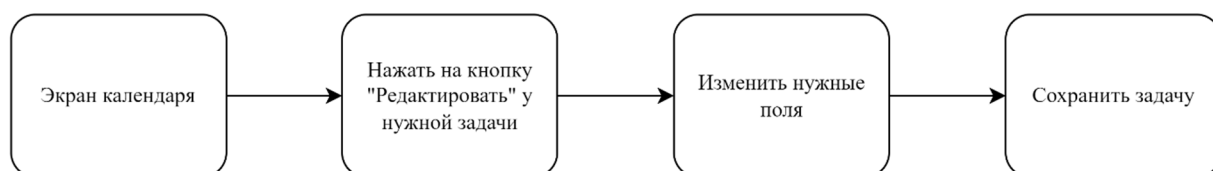
Рисунок 28 - Редактирование задачи
