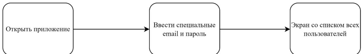
Рисунок 35 - Авторизация администратора
