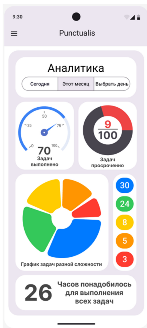
Рисунок 12 - Экран аналитики
