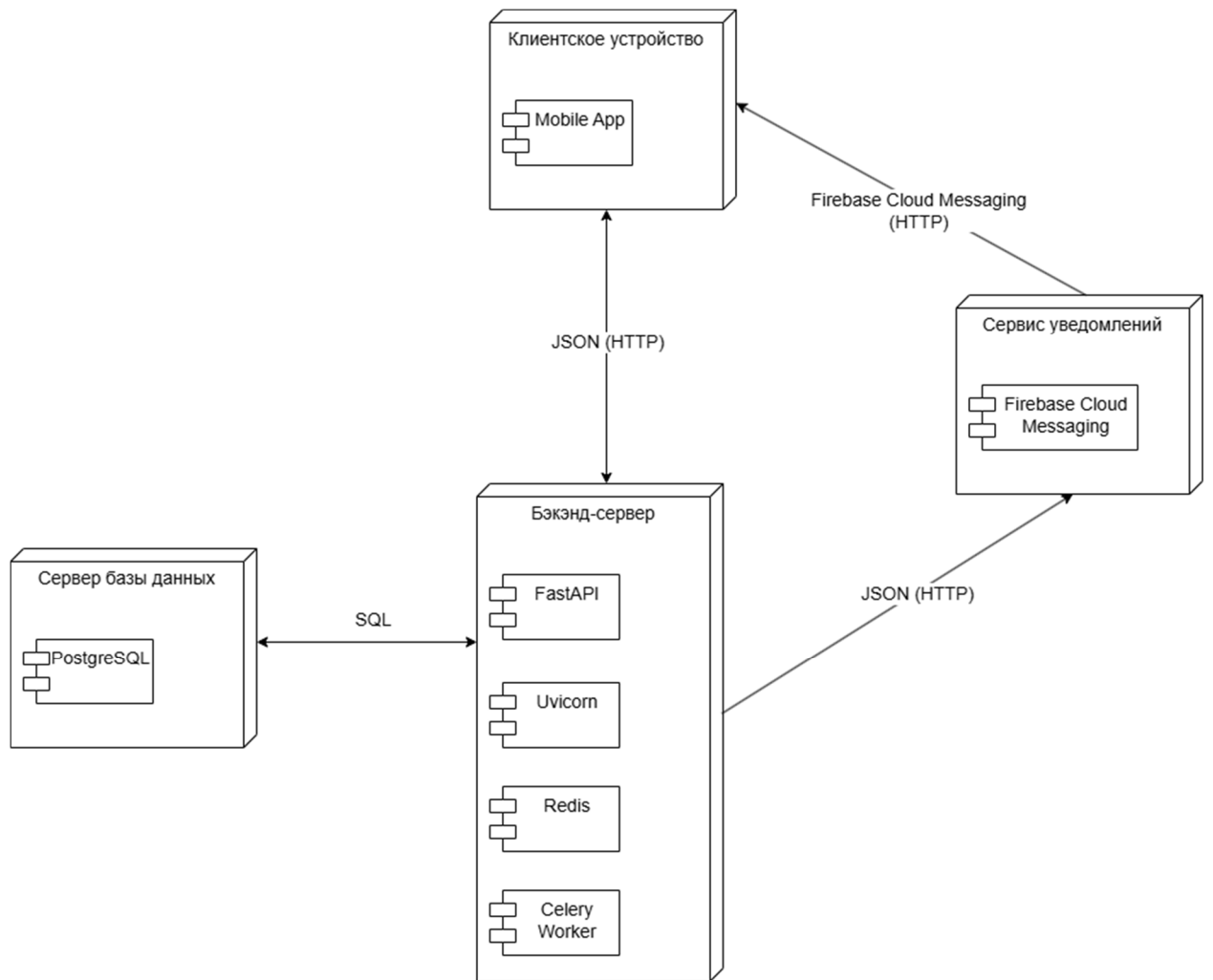
Рисунок 49 - Диаграмма развертывания
