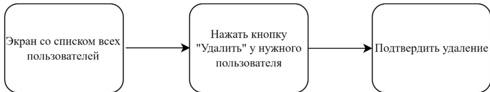
Рисунок 38 - Удаление пользователя
