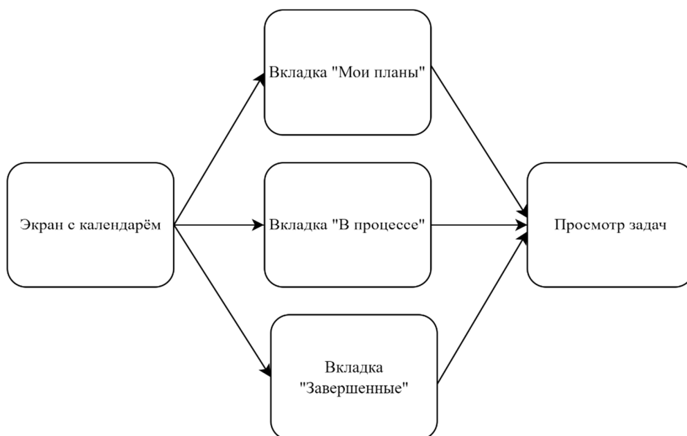
Рисунок 27 - Просмотр задач
