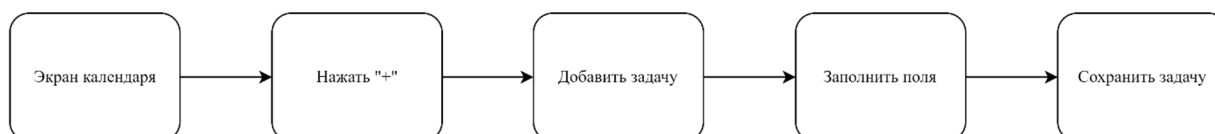
Рисунок 26 - Добавление задачи
