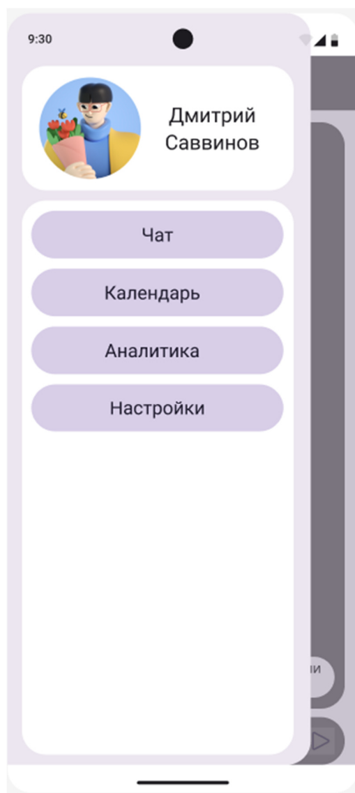
Рисунок 15 - Навигационная панель
