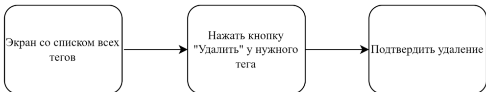
Рисунок 40 - Удаление тега
